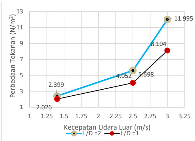
Gambar 5 grafik perbedaan tekanan static inlet dan outlet
