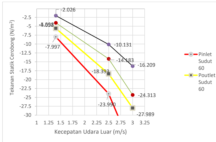
Gambar 3 grafik tekanan static inlet
