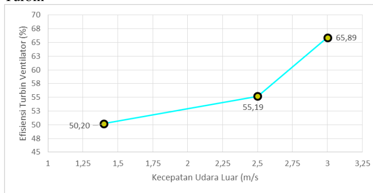
Gambar 7. Grafik Efisiensi Turbin
