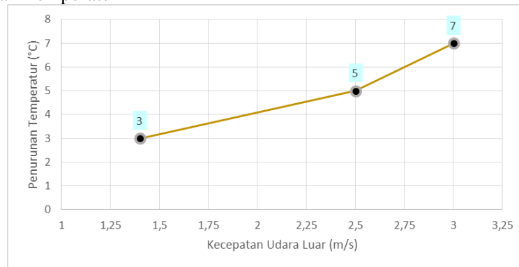
Gambar 4. Grafik Penurunan Temperatur
