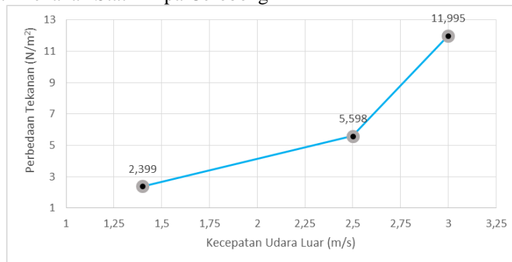
Gambar 2. Grafik Perbedaan Tekanan Statik Pipa Cerobong
