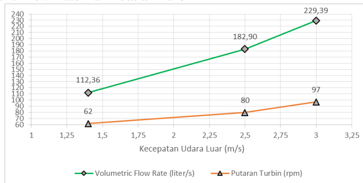
Gambar 3 Grafik Volumetric Flow Rate Dan Putaran Turbin
