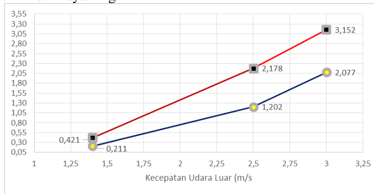
Gambar 6. Grafik Daya Listrik Dan Daya Angin
