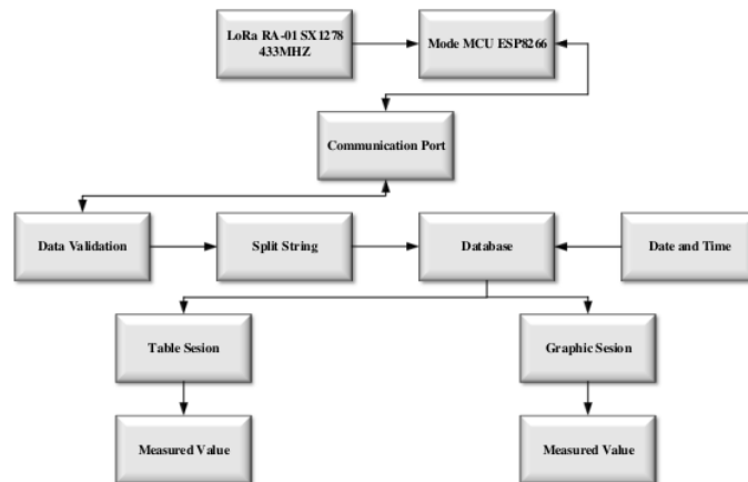
Gambar 3. Diagram Blok Keseluruhan Sistem.
