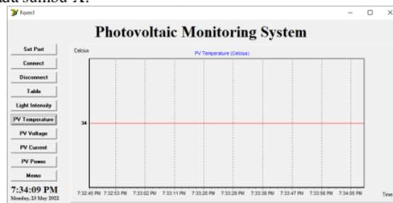
Gambar 13. Tampilan Grafik “PV Temperature”
