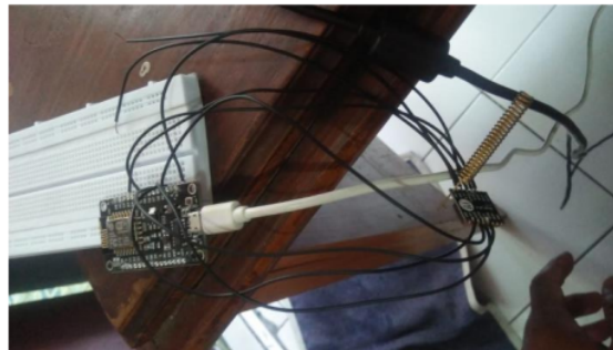
Gambar 4. Board LoRa dan Node MCU ESP8266 pada breadboard.
