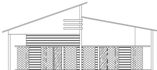
Gambar 21. Sumber: Dokumen Pribadi Tampak Depan
