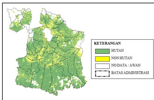
Gambar 4. Hasil Klasifikasi ARVI Citra Landsat 8 OLI/TIRS
