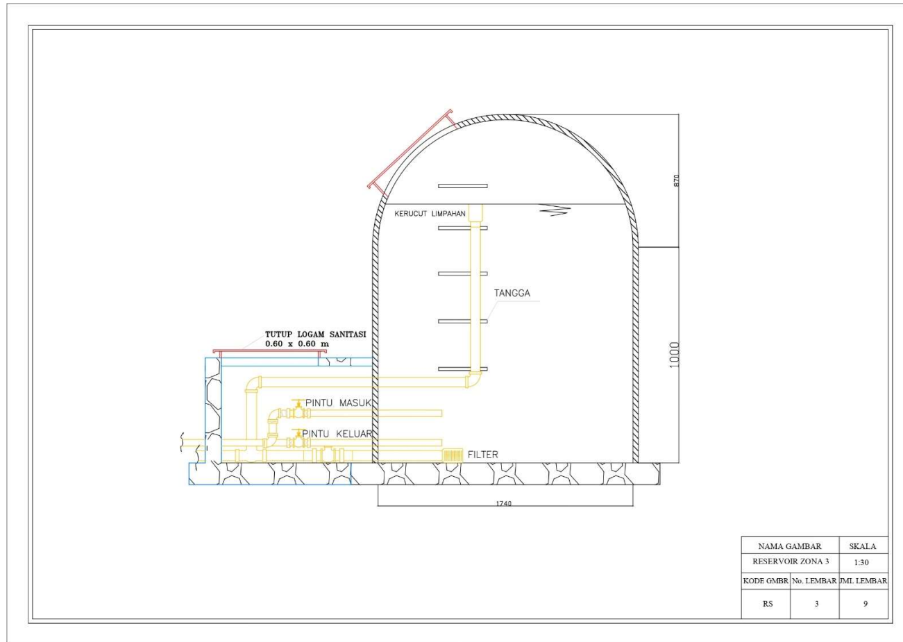
Gambar L. 3 Reservoir Zona 3
