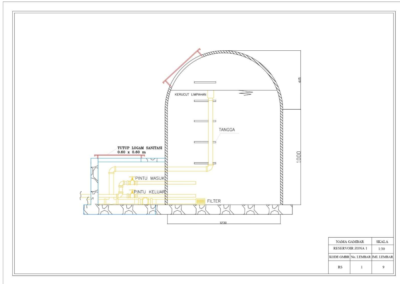
Gambar L. 1 Reservoir Zona 1
