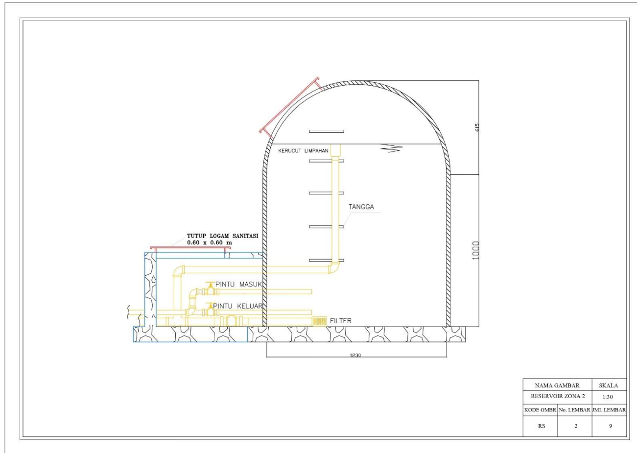
Gambar L. 2 Reservoir Zona 2
