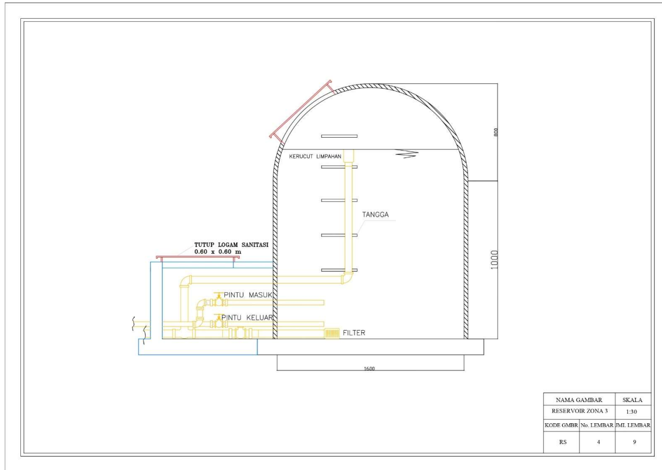
Gambar L. 4 Reservoir Eksisting Kapasitas 2000 M 3
