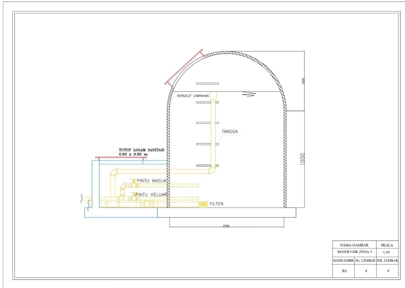
Gambar L. 6 Reservoir Eksisting Kapasitas 850 M 3
