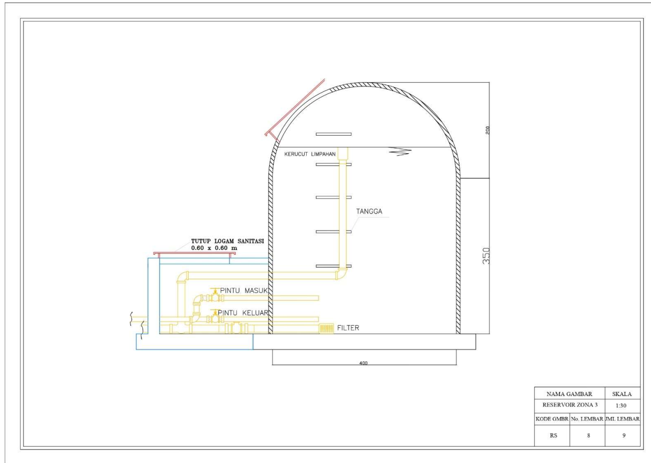
Gambar L. 8 Reservoir Eksisting Kapasitas 36 M 3
