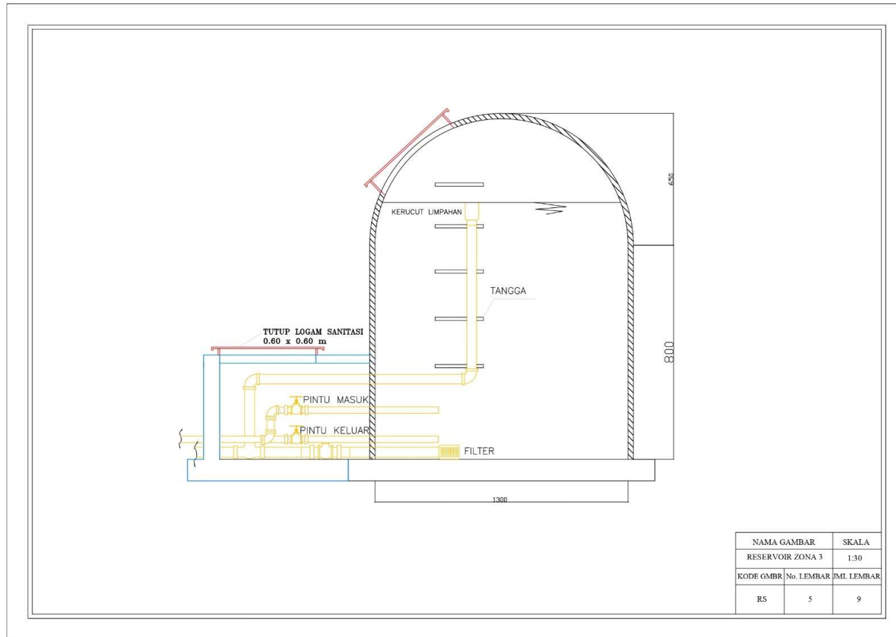
Gambar L. 5 Reservoir Eksisting Kapasitas 1000 M 3
