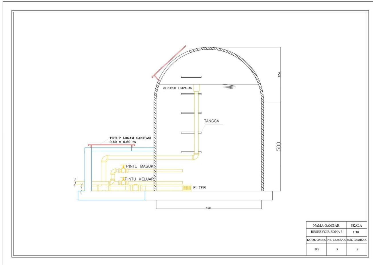
Gambar L. 9 Reservoir Eksisting Kapasitas 50 M 3
