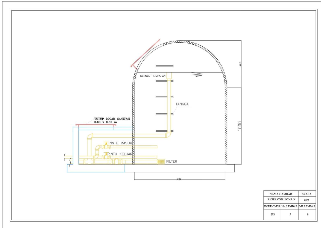
Gambar L. 7 Reservoir Eksisting Kapasitas 500 M 3
