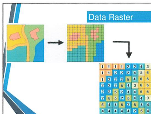
Gambar 2.6 Peta Raster
