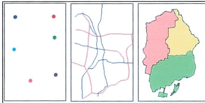
Gambar 2.5 Peta Vektor
