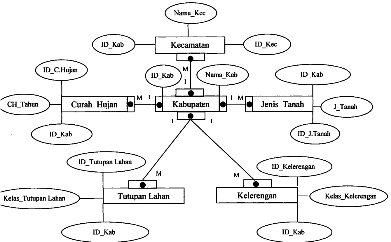
Gambar 3.16 Diagram ER
